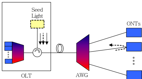
(그림 10) Colorless WDM-PON 구조
