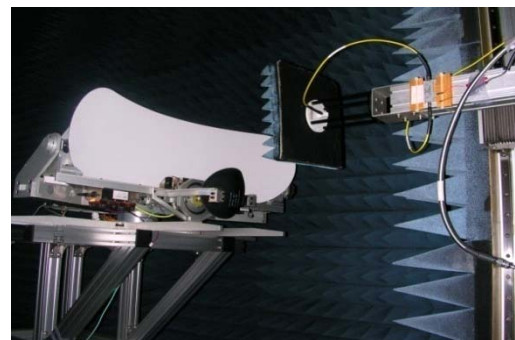
(그림 8) 무반향실 내에서의 안테나 성능 측정
