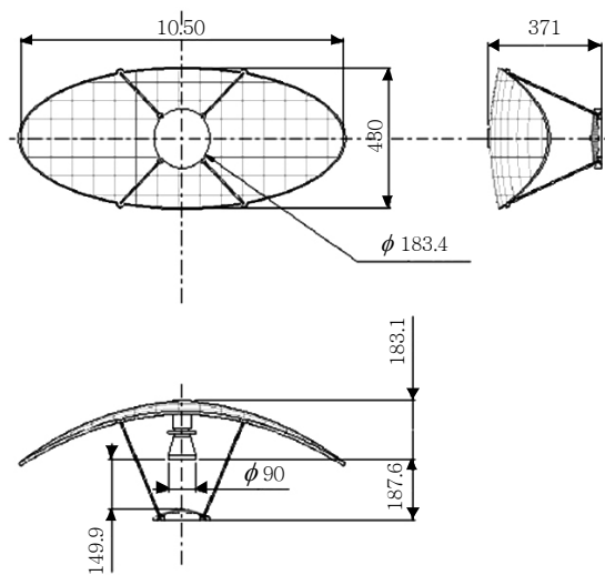
(그림 6) Alcatel사의 안테나 설계 결과
