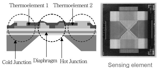
<자료>: GE Sensing사 (그림 5) 써모파일 적외선 센서의 구조(좌) 및 칩 사진(우)
