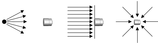
(그림 11) 음향 센서의 응용별 유형: Free-field(좌), Pressure-field(중), Random-incident-field(우)
