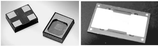
(그림 14) Knowles Acoustics사의 MEMS형 초음파 센서(좌)와 마쓰시타사의 나노 결정 Si 초음파 발생기(우)
