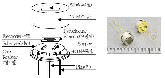
<자료>: Murata사 (그림 6) 박막형 초전 센서의 구조(좌) 및 제품 사진(우)
