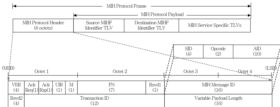
(그림 4) IEEE 802.21 MIH 프로토콜 프레임
