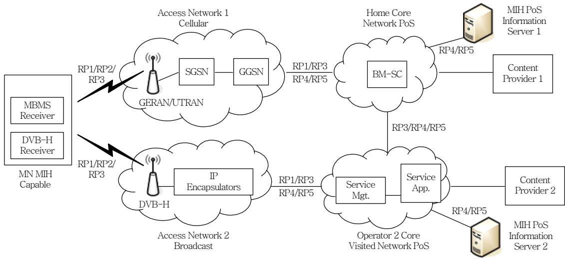
(그림 8) IEEE 802.21 TGb의 로밍 형태 네트워크 모델
