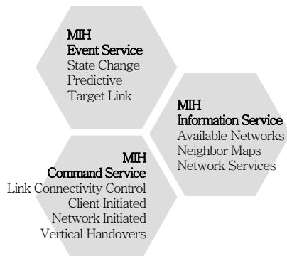
(그림 2) IEEE 802.21 MIHF 서비스
