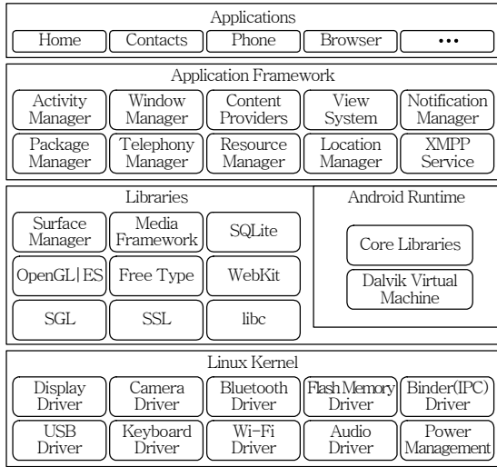
(그림 9) 안드로이드 소프트웨어 플랫폼 구조
