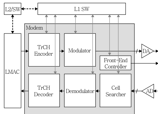
(그림 5) 3GPP 단말 모뎀 구조도
