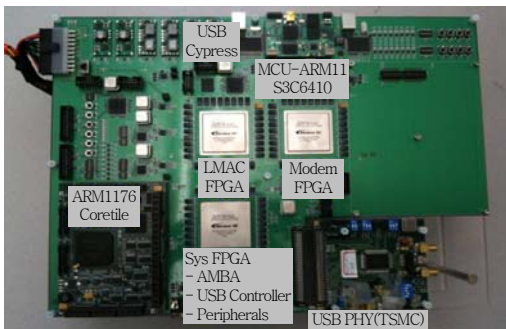
(그림 7) LTE Modem Soc 플랫폼 구조도
