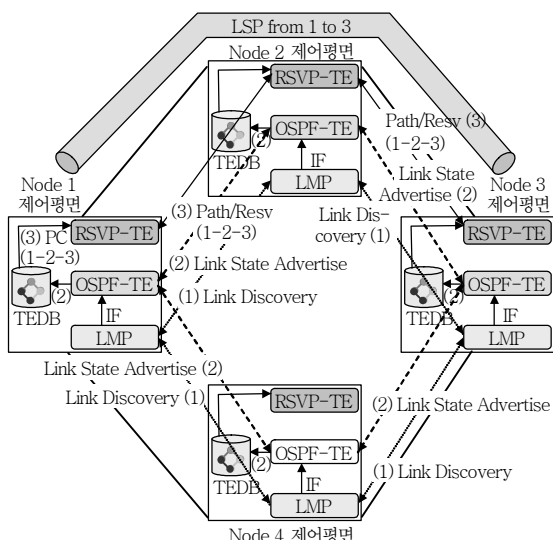
(그림 6) GMPLS 동작 절차
