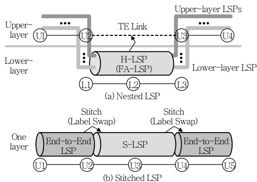
(그림 8) Nested LSP vs. Stitched LSP
