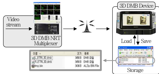
(그림 8) 반복 콘텐츠를 이용한 비실시간 스테레오스코픽 비디오 서비스 시스템 및 실험 결과
