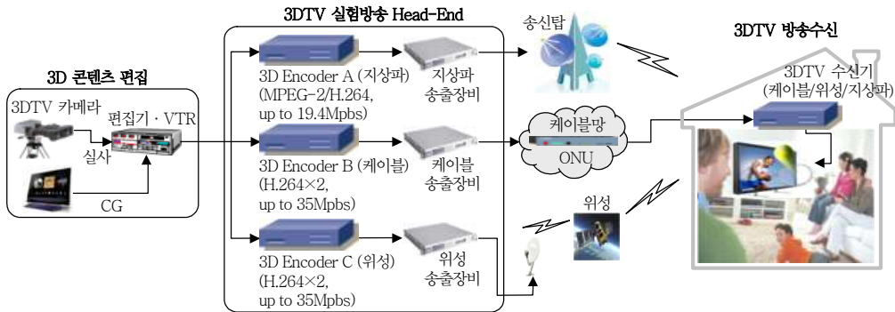
(그림 4) 실험 방송 시스템 구성도
