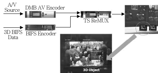
(그림 6) 지상파 DMB 3D 데이터 서비스 방송 실험
