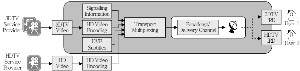
(그림 2) DVB-3DTV 서비스 범위[4]
