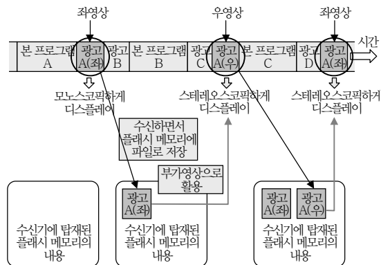
(그림 7) 반복 콘텐츠를 이용한 비실시간 스테레오스코픽 비디오 서비스 시나리오
