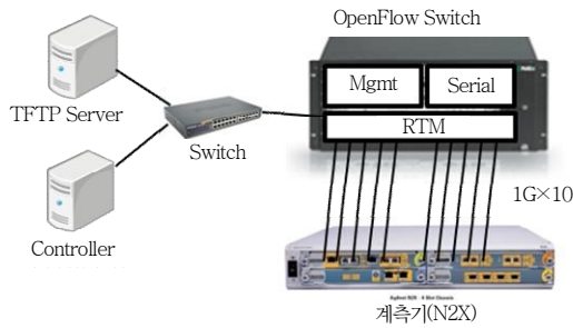
(그림 8) OpenFlow 시험망 구성도
