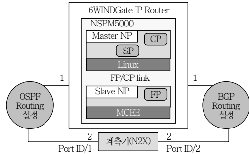
(그림 9) Legacy IP Router 시험 구성도
