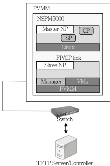
(그림 7) PVMM 시험 구성도
