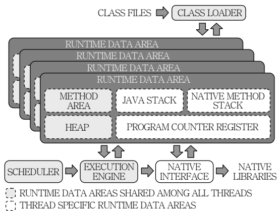
(그림 4) PVMM 구조
