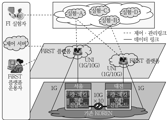
(그림 10) FiRST 플랫폼 KOREN 연구개발망 적용
