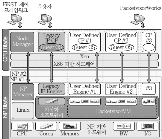
(그림 3) FIRST의 S/W 구조
