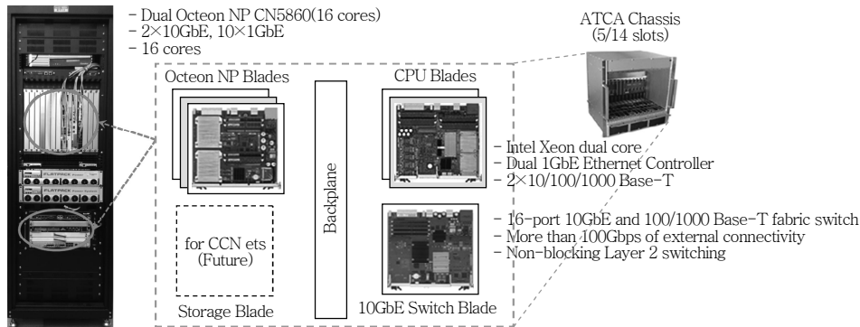
(그림 2) FIRST의 H/W 구조
