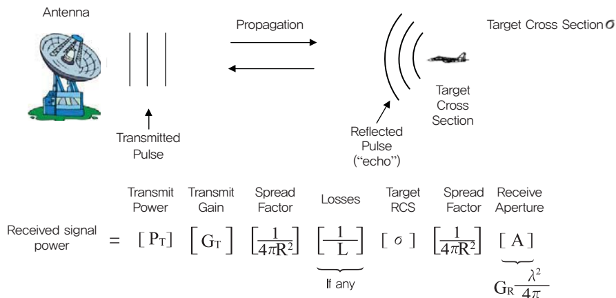
(그림 1) 레이다의 원리와 레이다 방정식
