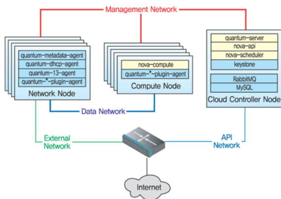
(그림 4) OpenStack 네트워크 구축 모델
