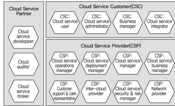
<그림1> CT-CCRA의 Role과 sub-role[12]
