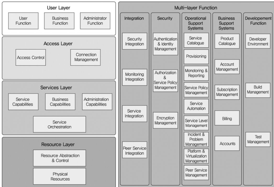
(그림 2) CT-CCRA의 계층 구조와 기능 component[12]
