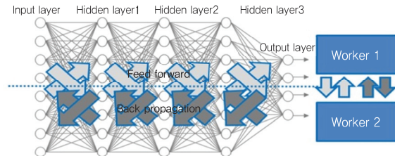
(그림 3) 입력 피처 별 모델 분할([9]의 재구성)
