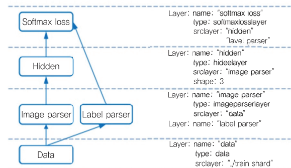
(그림 8) NeuralNet 형상[15]
