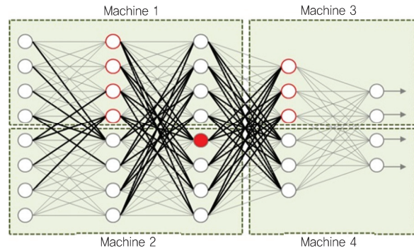
(그림 6) 모델 병렬 처리 예
