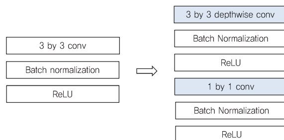
(그림 8) MobileNet-v1[51] 기본 구조
