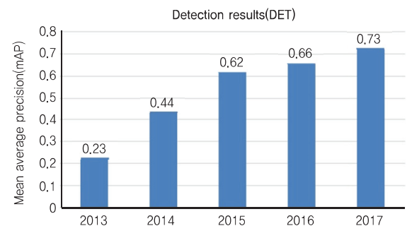
(그림 2) ILSVRC 객체 검출 성능 변화
