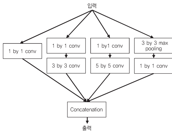
(그림 4) Inception 모듈 기본 구조[22]
