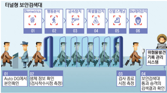
(그림 6) 인천공항의 터널형 보안검색 절차 개념도
