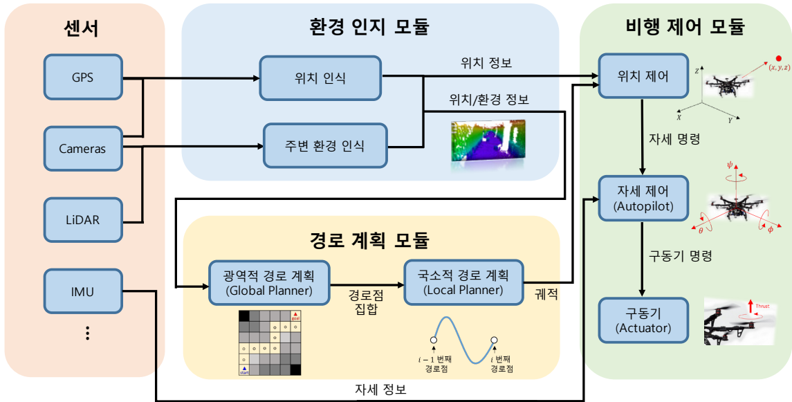
그림 1 무인 비행체의 자율 비행을 위한 환경 인지 및 경로 계획 구성도
