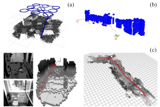
그림 2 SLAM 기반 환경 지도 형태[1]: (a, c) 3차원 포인트 클라우드 맵, (b) occupancy grid 맵 출처 C. Kanellakis and G. Nikolakopoulos, "Survey on Computer Vision for UAVs: Current Developments and Trends," J. Intell. Robot. Syst., vol. 87, no.1, 2017, pp. 141-168. CC BY 4.0
