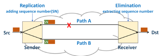
그림 4 802.1CB FRER 동작[9]
