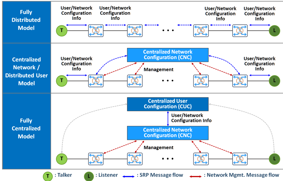
그림 5 802.1Qcc TSN 설정 모델[10]
