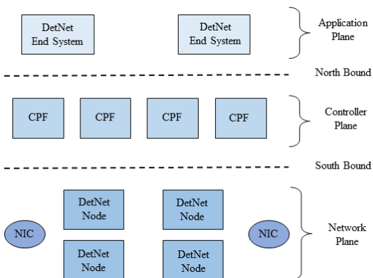
그림 6 DetNet 평면 및 인터페이스[12]
