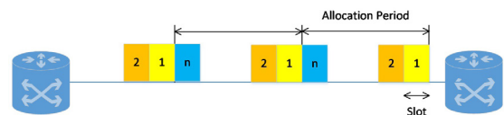
그림 10 Flexilink 프로토콜의 동기식 전송방식[30]
