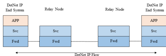
그림 7 DetNet IP 데이터 평면[15]
