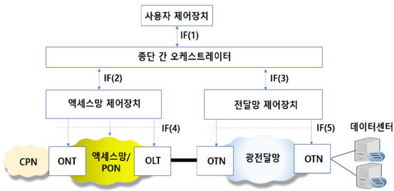
그림 9 중단 간 초저지연 제어 구조 예
