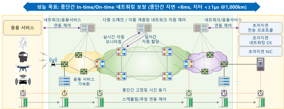
그림 1 초정밀 네트워크 개념도
