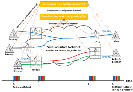
그림 2 IEEE 802.1 TSN 네트워크 구성[5]
