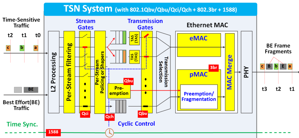
그림 3 802.1Qbv/Qch/Qbu 기반 TSN 포워딩[7,8]
