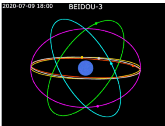
그림 3 BDS 위성군 배치현황
