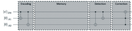
그림 5 양자 오류 정정 회로 순서. 부호화-결폴립-복호화-회복(오류 정정)-상태 측정 과정을 거침
