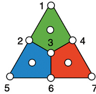
그림 3 ((7,1,3)) Steane code 구조 (순서가 매겨진 노드가 데이터 큐비트를 의미하고, 그렇지 않은 노드는 신드롬 큐비트를 의미함)
