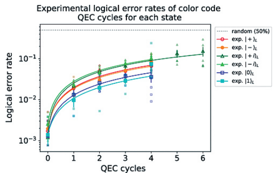
그림 4 QEC 사이클을 반복하여 측정한 logical state에 대한 오류율과 시뮬레이션 결과의 비교
