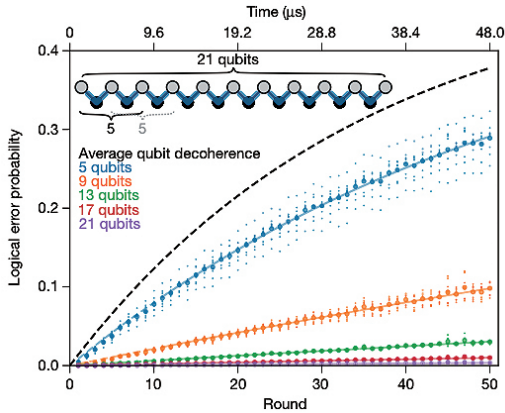
그림 2 Repetition code의 Data Block 길이 증가에 따른 Logical Error Rate 감소
