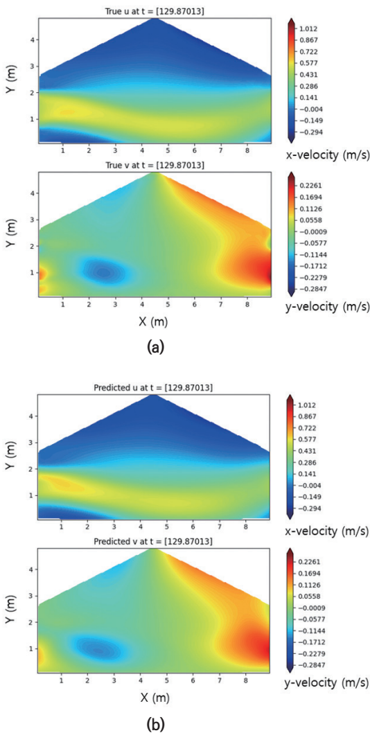
그림 4 PINN 기반 온실 내부 유동 해석 결과 예시: (a) CFD 기반 유동해석 결과, (b) PINN 기반 유동해석 결과
