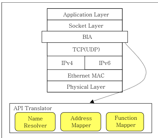
(그림 4) BIA 구조
